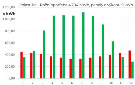
Roční struktura spotřeby el. energie po instalaci HFVE
